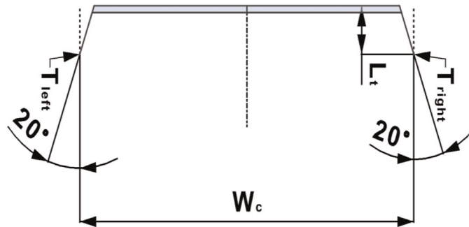
Figuur 2 3D-omhulling
