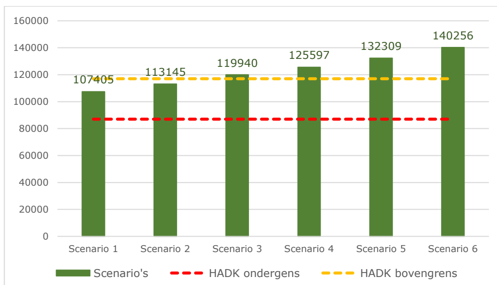
Figuur 3: Scenario's aantal EV-nieuwverkoop in 2024
